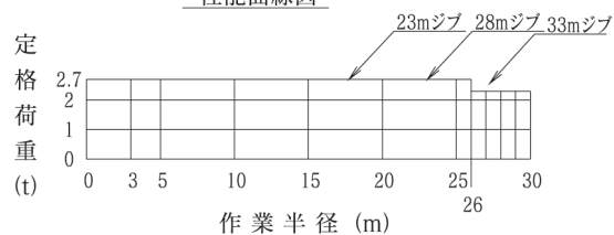
性能曲線図
