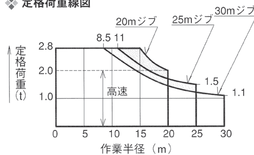
◆ 定格荷重線図
