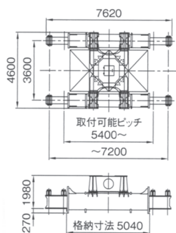
伸縮架台仕様 (オプション)
